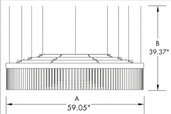
SF-150-055-016-03
